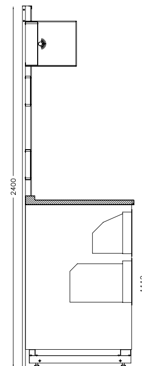
RETRO BANCO M. CAFFÈ CON ALZATA ESPOSITIVA MODELLO: GLAMOUR - EASY - FASHION BAR STATION WITH DISPLAY UPPER PART
