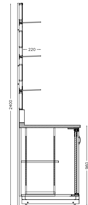
RETRO BANCO CON ALZATA 3M MODELLO: GLAMOUR - EASY - FASHION BAR STATION STRUCTURE 3M
