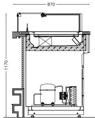
TAVOLA FREDDA VENTILATA MODELLO: EASY - FASHION VENTILATED BUFFET
