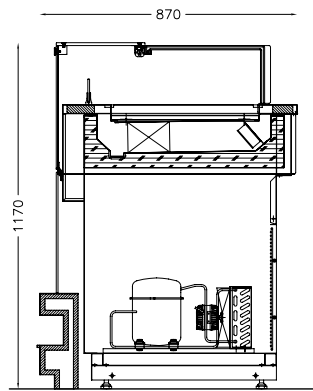
TAVOLA FREDDA VENTILATA MODELLO: GLAMOUR VENTILATED BUFFET
